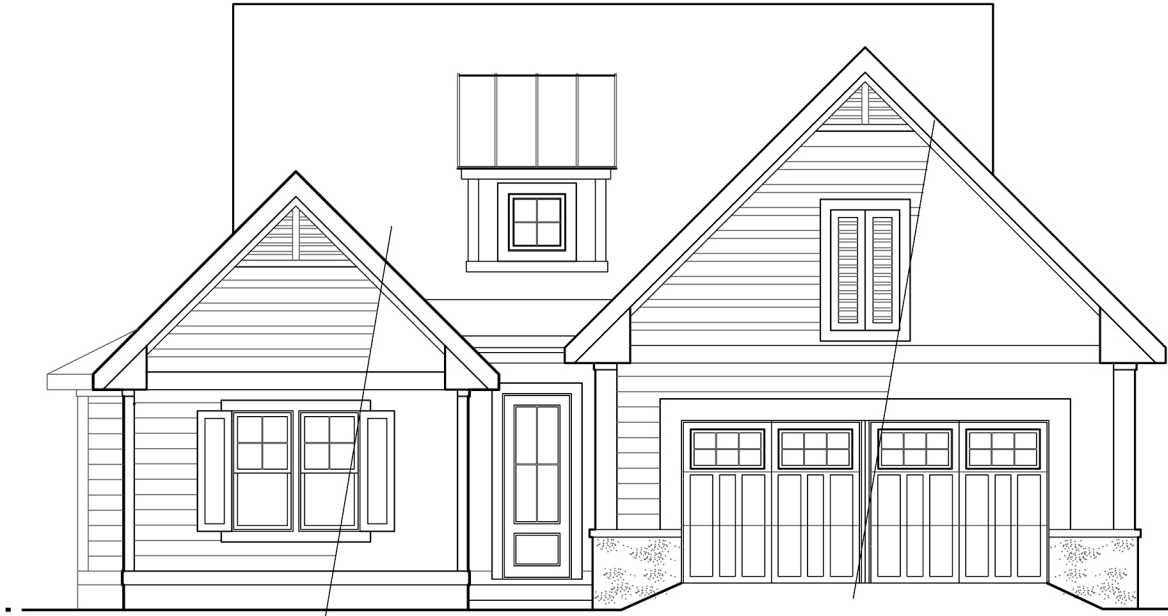
Elevation A
